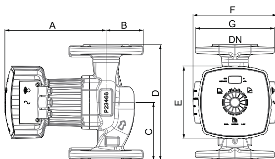
Rys. 3: Agregat pompowy z przyłączem kołnierzowym
