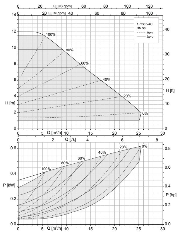
Calio 50-150 \Delta p -v, \Delta p -c
