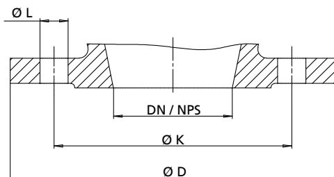
Rys. 6: Wymiary kołnierzy Etablo SYT / Etaline SYT
