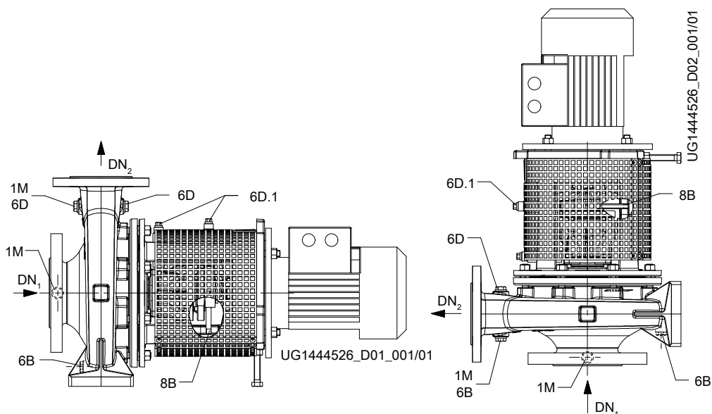
Rys. 7: Etabloc SYT wersja przyłącza wg rodzaju ustawienia
